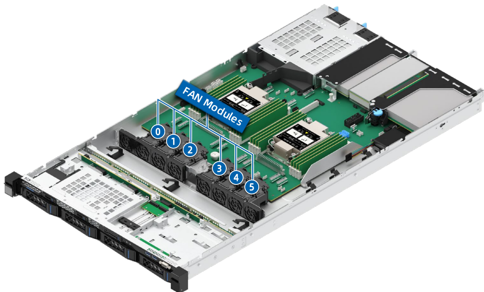
图 5-18 风扇模组位置
