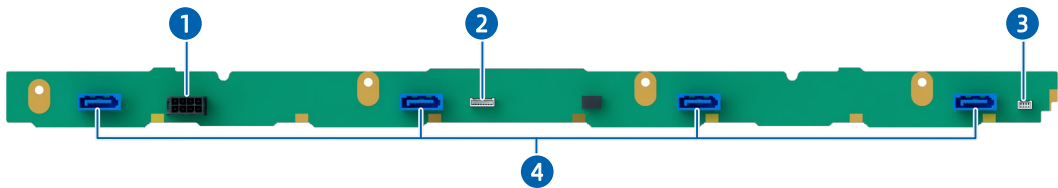
图 5-21 4 × 3.5 英寸硬盘背板 (SAS/SATA)
