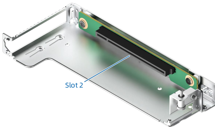
图 5-15 LP PCIe 转接卡模组
