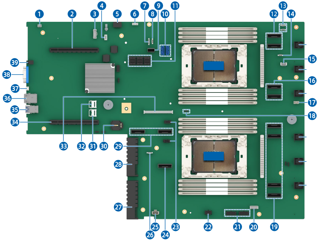
图 5-20 主板
