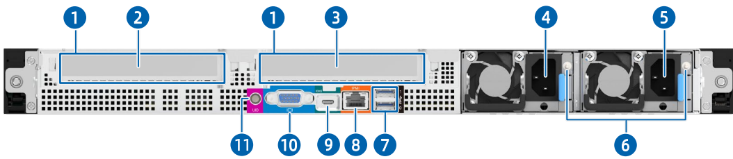
图 5-3 后视图-2 × PCIe
