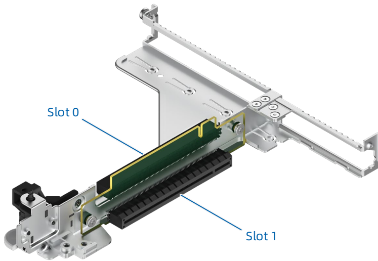
图 5-14 蝴蝶卡 PCIe 转接卡模组
