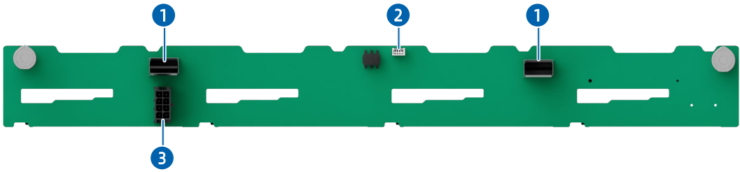
图 5-23 8 × 2.5 英寸硬盘背板 (SAS/SATA)
