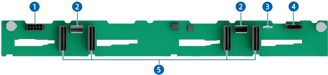
图 5-27 8 × 2.5 英寸硬盘背板 (SAS/SATA/NVMe)
