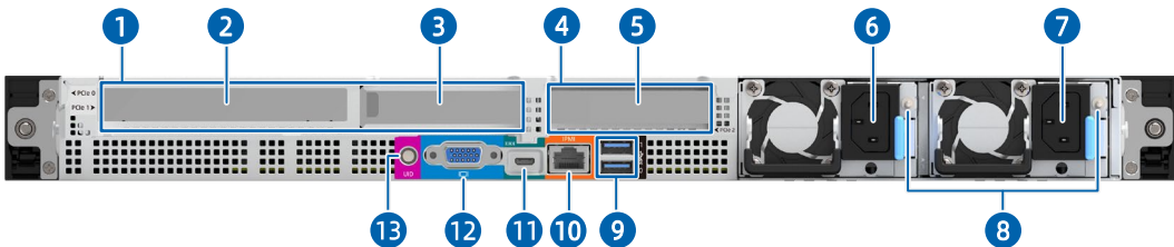
图 5-4 后视图-3 × PCIe
