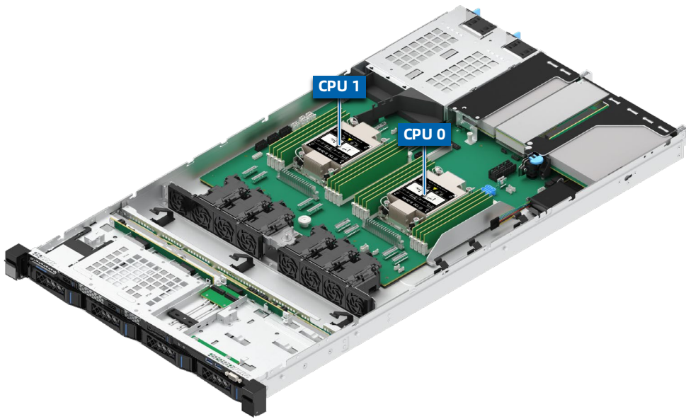
图 5-5 处理器位置
