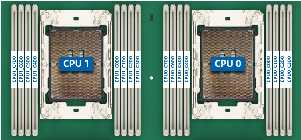
图 5-7 内存插槽位置
