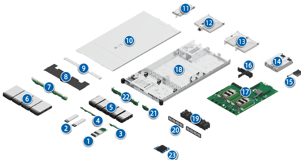
图 3-1 NF5170-M7-A0-R0-00 物理结构
