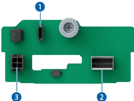
图 5-25 2 × 2.5 英寸背板 (SAS/SATA)
