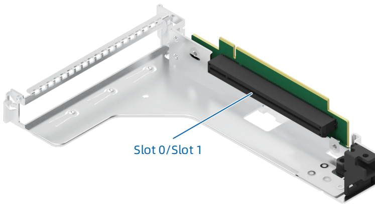
图 5-16 FH PCIe 转接卡模组
