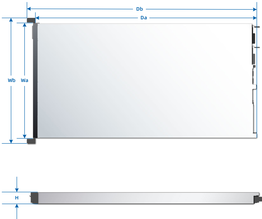
图 6-1 主机尺寸
