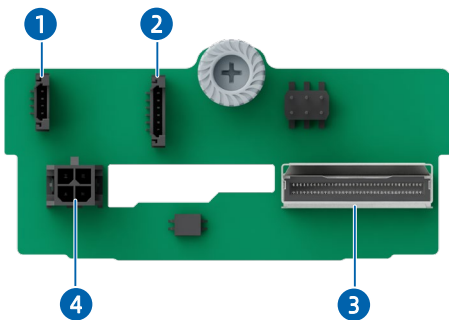
图 5-28 2 × 2.5 英寸硬盘背板 (NVMe)
