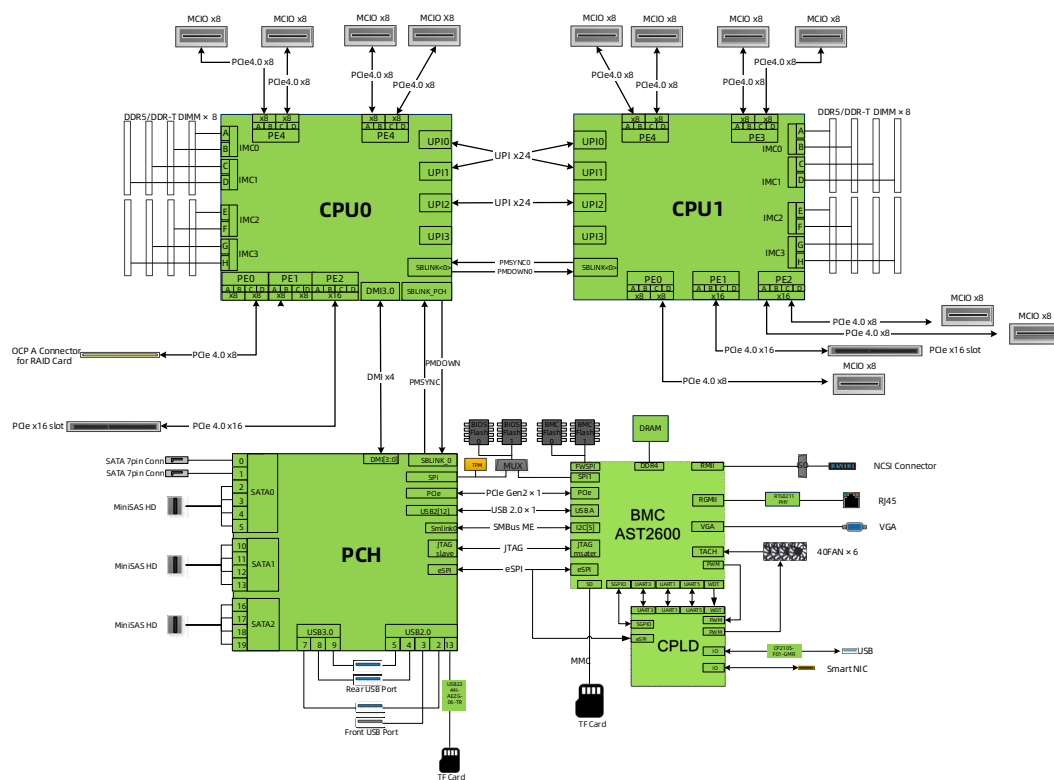
图 4-1 NF5170-M7-A0-R0-00 逻辑结构
