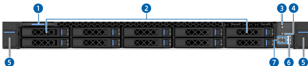
图 5-2 前视图
