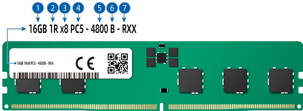
图 5-6 内存标识
